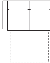
41 (P/L) – 2-křeslo s područkou rozkládací 161 (170*) × 98 (230**)/ v. 83 (ložná plocha 128 × 190/ v. 44)
