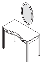
Stolek toaletní - bez zrcadla LTS (100 x 70 x 50)
